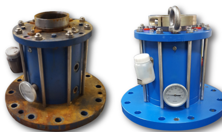
EXEMPLE DE RECONDITIONNEMENT D'UN BOÎTIER D'AGITATION
