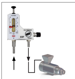
LATTYlub Flowcontrol 1 Contrôle le débit
