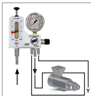
LATTYlub Flowcontrol 3 Contrôle le débit et la pression
