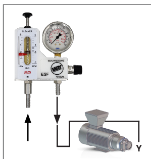
LATTYlub Flowcontrol 2 Contrôle le débit et indique la pression
