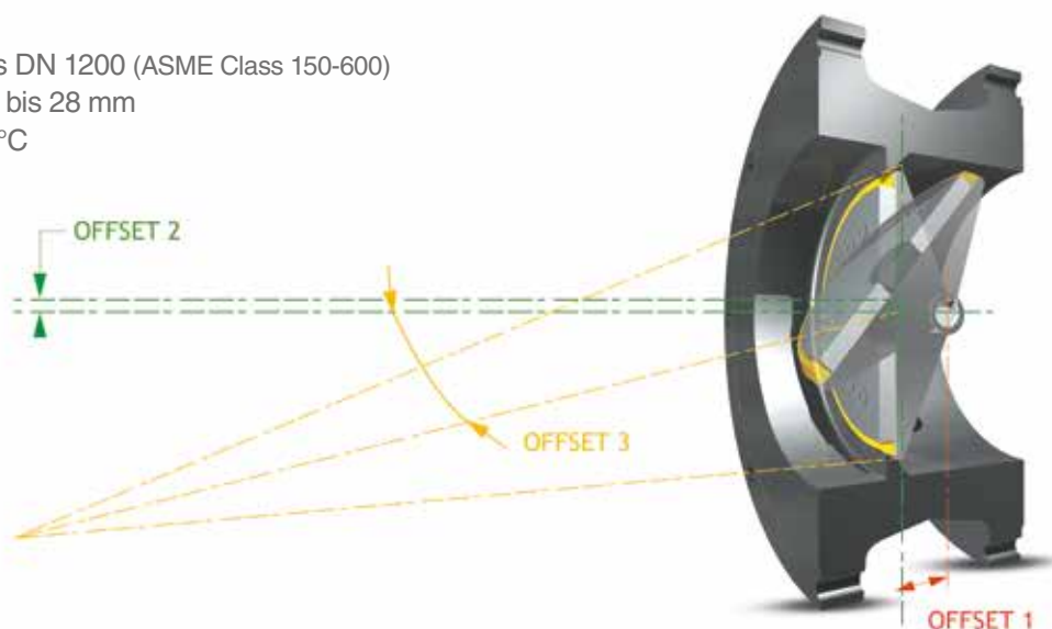
Variante 2 : Dichtung im Ventilkörper, Dichtungsfläche auf der Innenseite der Dichtung
