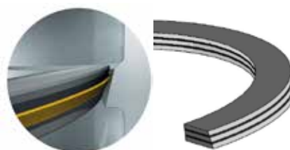
Variante 1 : Dichtung auf dem Schließglied, Dichtungsfläche auf der Außenseite der Dichtung
