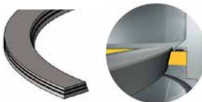
Variante 2 : Dichtung im Ventilkörper, Dichtungsfläche auf der Innenseite der Dichtung
